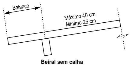
Beiral sem calha
