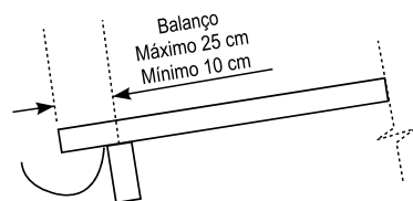
Beiral com calha
